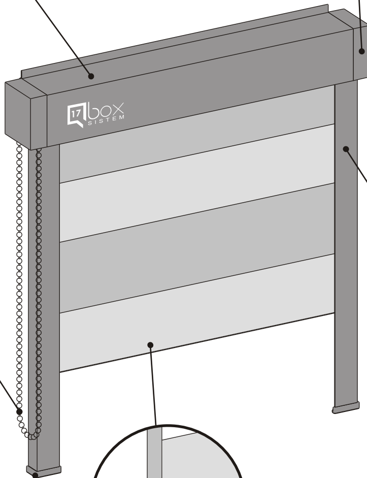
Profil contragreutate din aluminiu Culori: alb, negru
