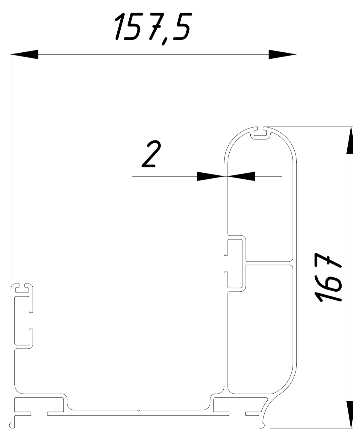
POS-2 4,279 kg/m
