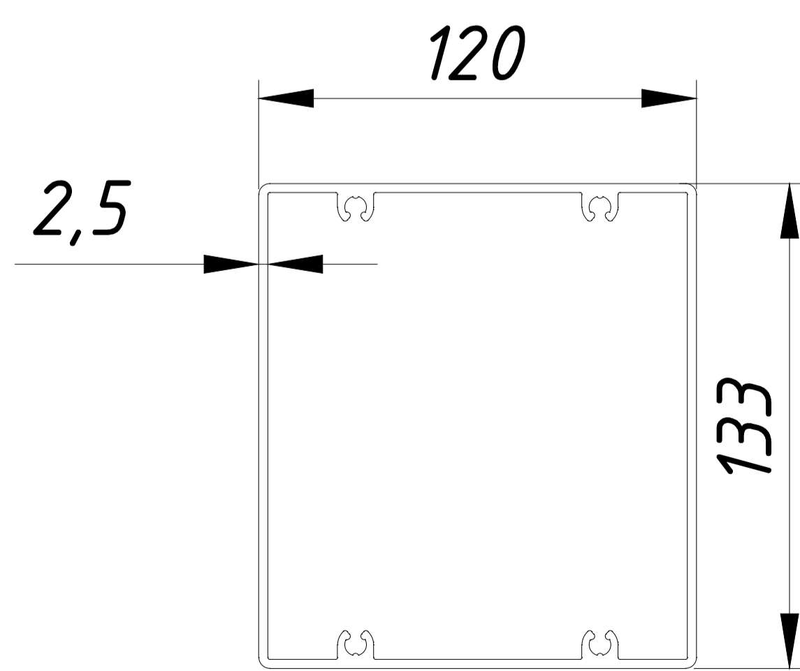
POS-4 3,807 kg/m
