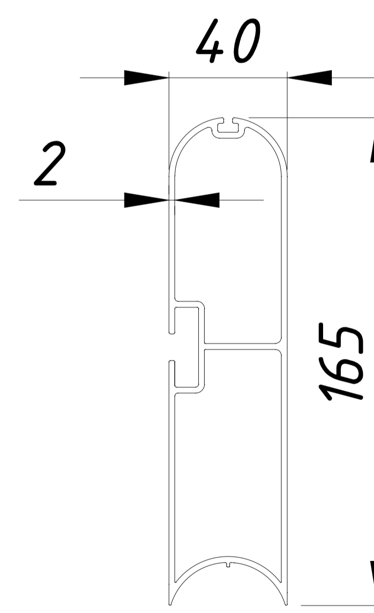
POS-3 2,54 kg/m
