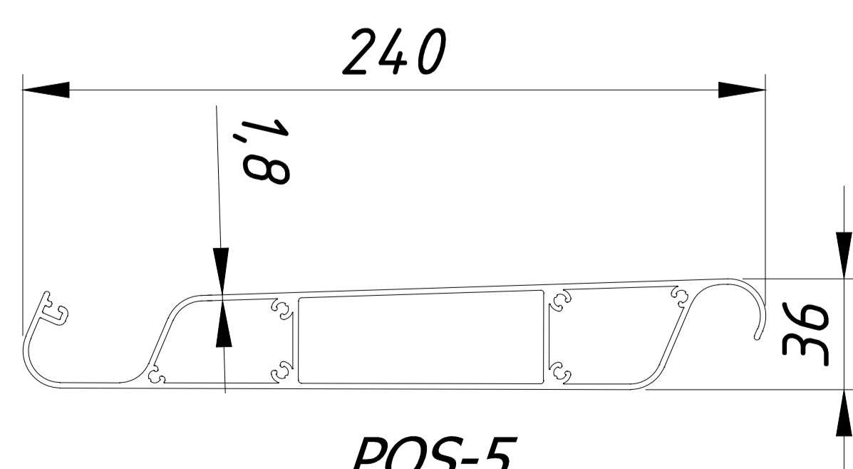
POS-5 3,13 kg/m
