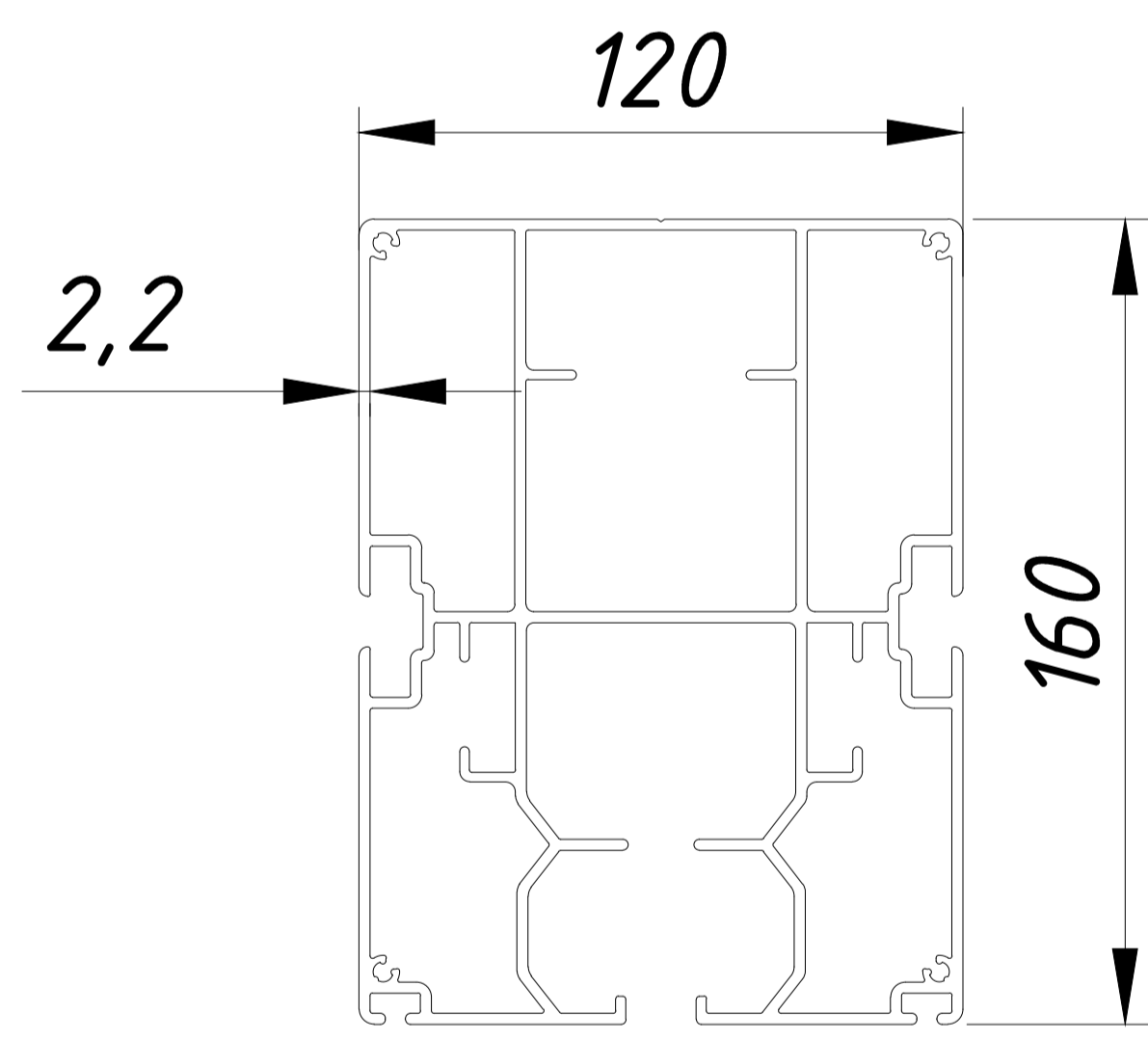
POS-1 6,88 kg/m
